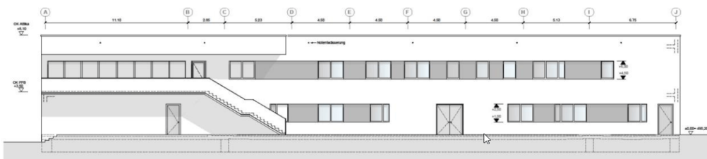
Ansicht Süden
